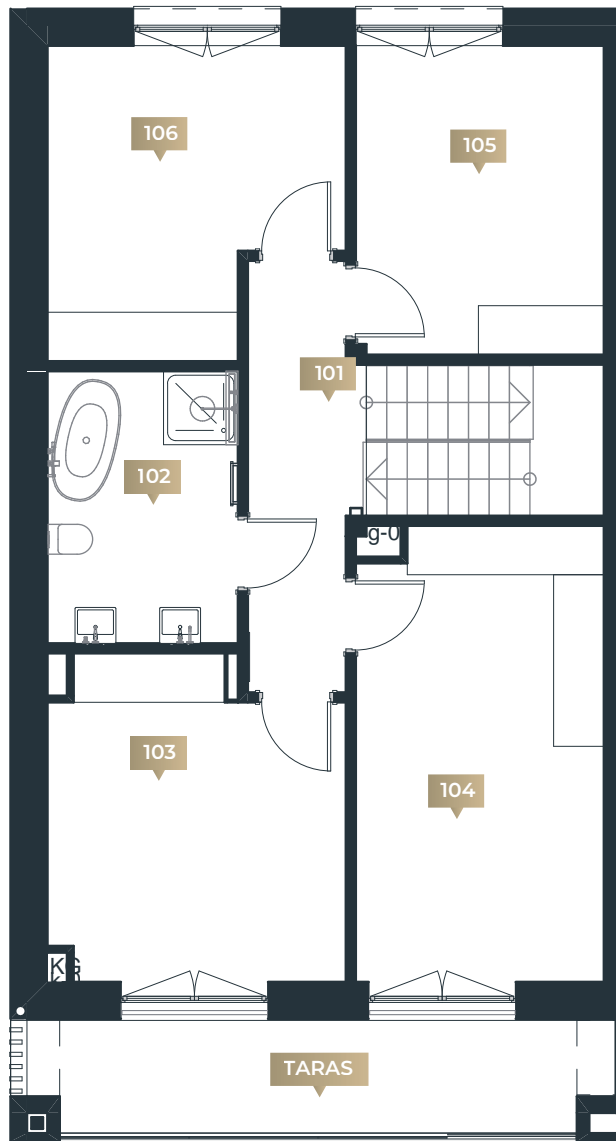
RZUT PIĘTRA
