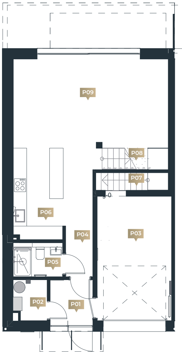
RZUT PARTERU
